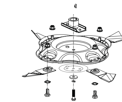
Quadcut® geležtė
