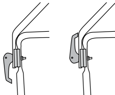
Posição bloqueada por altura de expedição.
